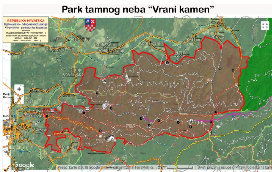
Slika 1 Geografski prikaz Međunarodnog parka tamnog neba Vrani kamen
