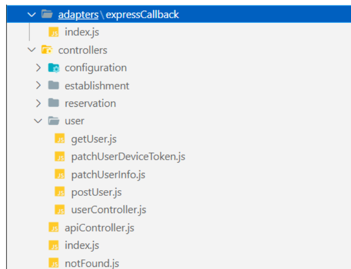
Slika 8. Prikaz strukture adaptera sučelja te kontrolera
