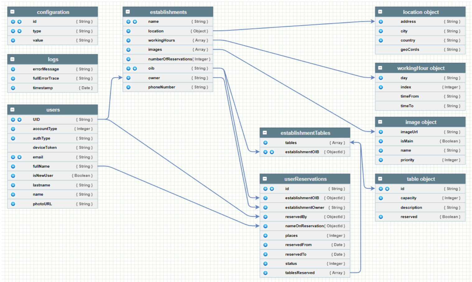
Slika 12. Struktura baze
