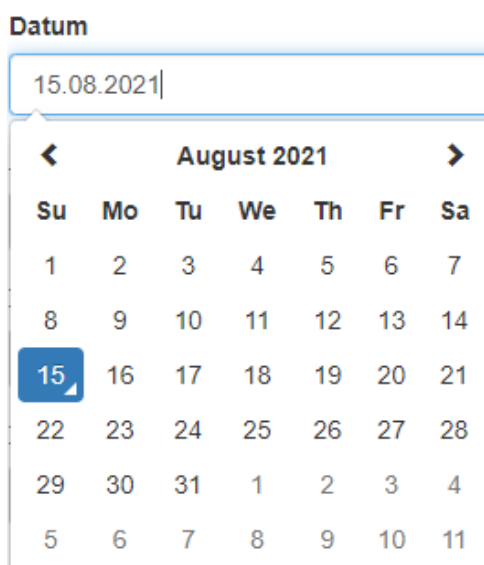
Slika 20. DateTimePicker
